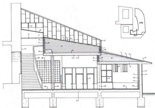
Sección, conexión con el edificio existente. Section, connection with the existing building.
