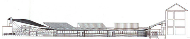
Alzado Patio. Elevation Patio.
